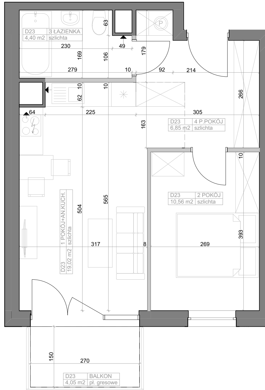
SCHEMAT BUDYNKU
