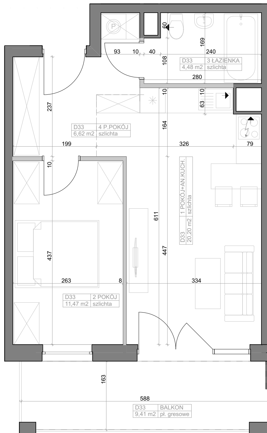
SCHEMAT BUDYNKU
